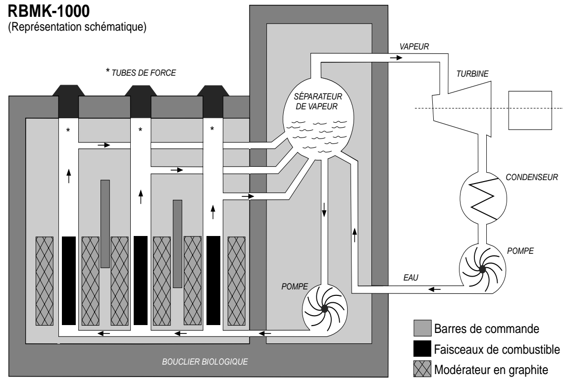
Figure 2. Le réacteur RBMK
