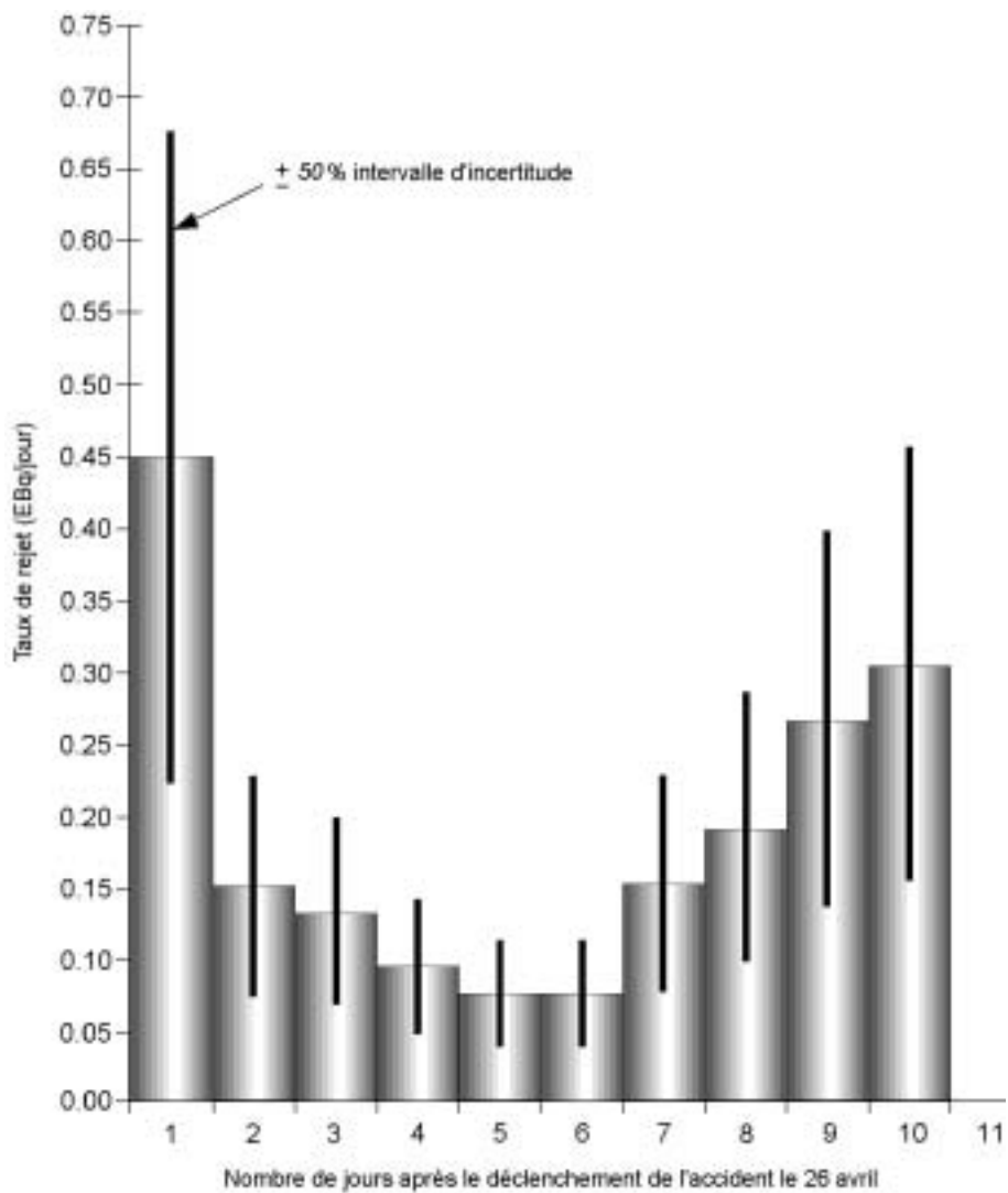
Figure 3. Taux de rejet quotidien de substances radioactives dans l'atmosphère (IA86a, version modifiée)
