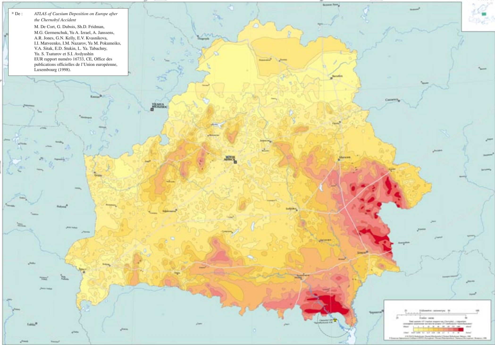
Figure 4. Dépôt de ^{137}\text{Cs} au Bélarus*
